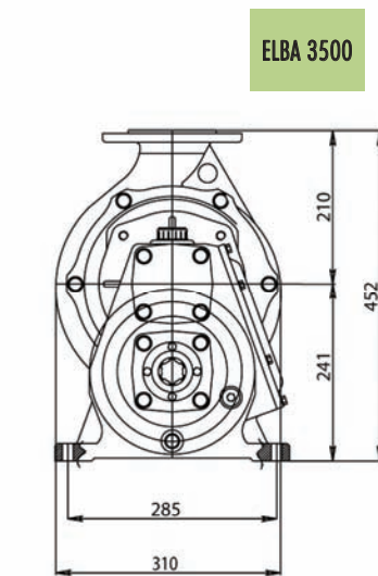
Dimensions de la centrifugeuse BP ELBA
