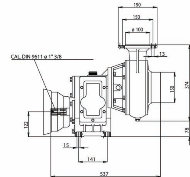
Abmessungen BP Zentrifugalpumpe ELBA
